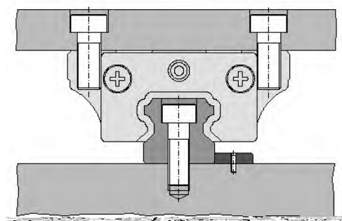
Piastra laterale Side plate
